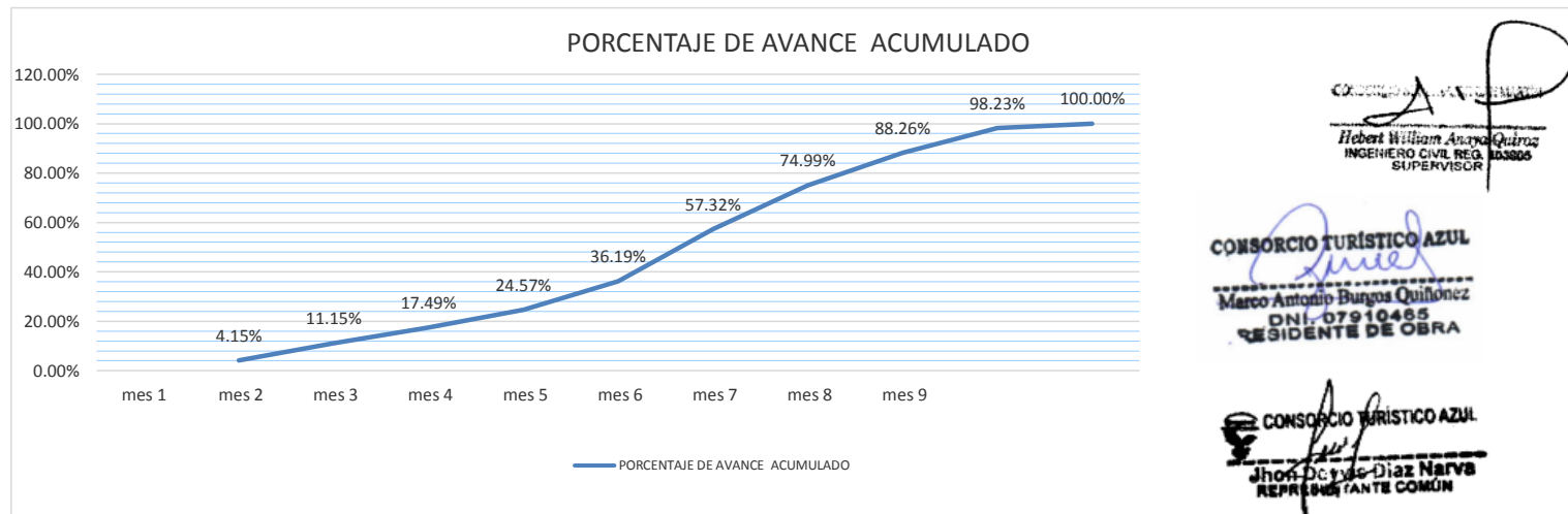
CURVA "S"
